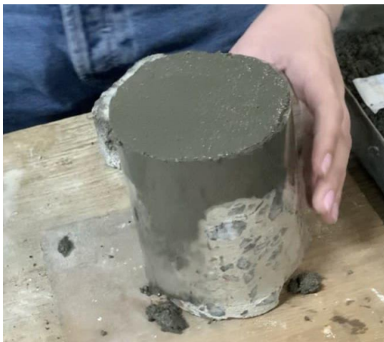
Рис. 8. Підготовка кернів до випробувань: а – очищення поверхні, б – нанесення ремонтної суміші Maregrout Thixotropic
